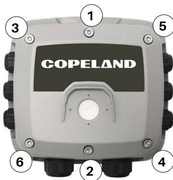
Schéma de serrage
